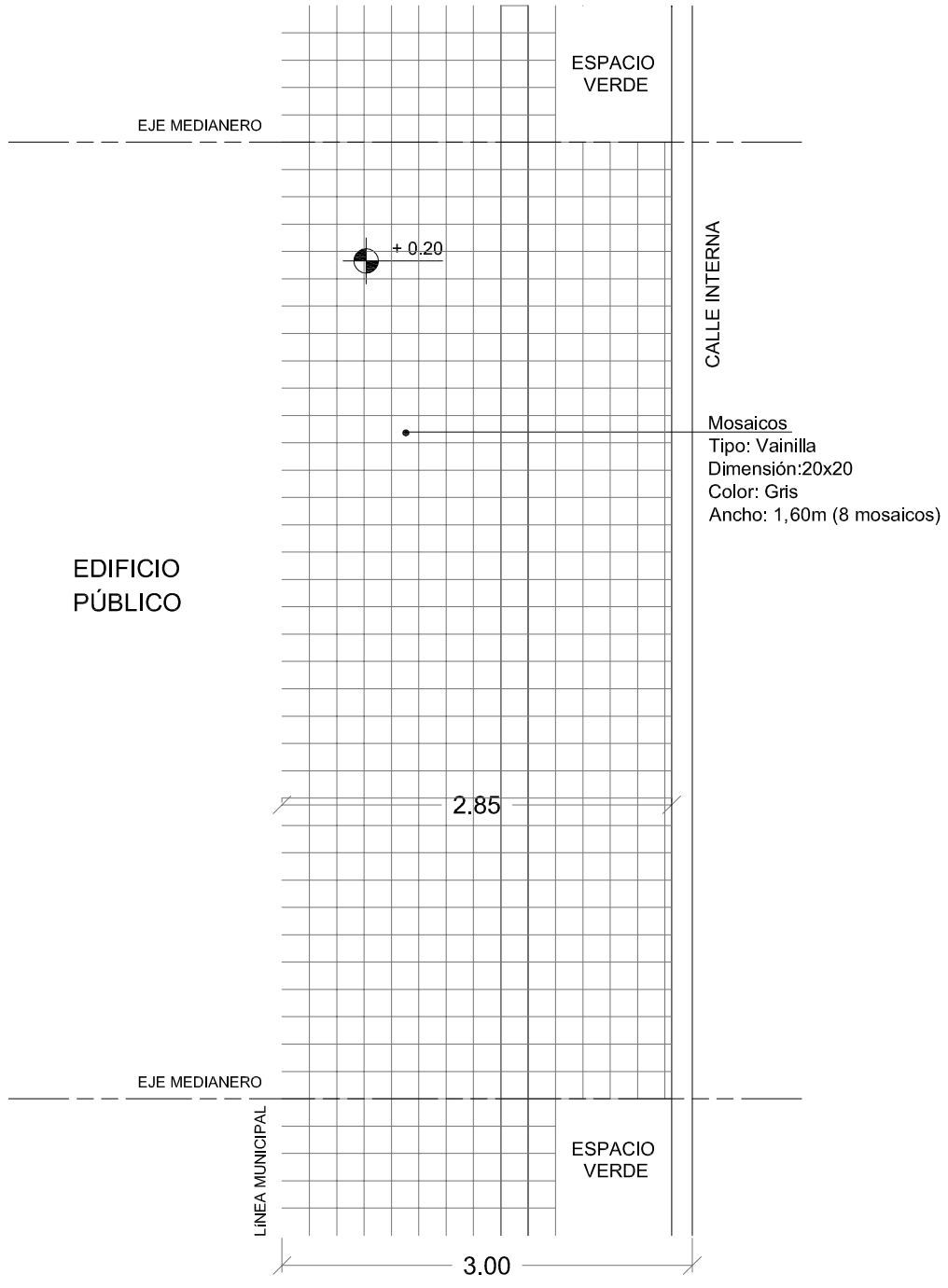
PLANTA / Esc. 1:50 Esquema: veredas en Calles internas
